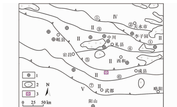
图1 那家坝区域构造略图
