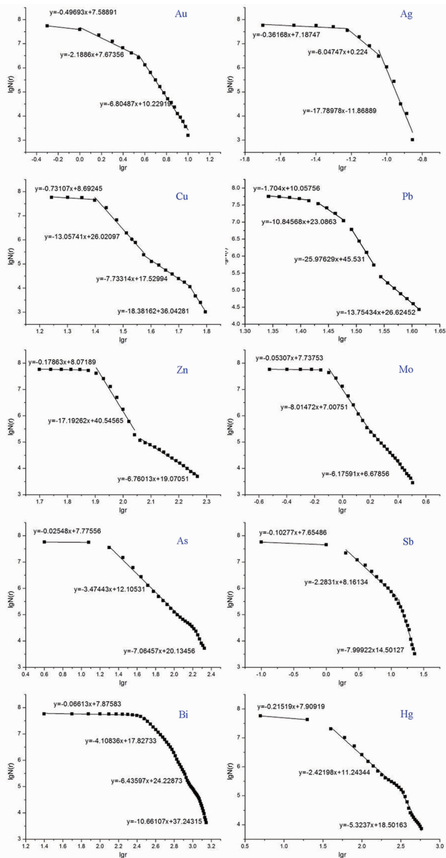
图 4 10 种元素的含量—面积关系图与拟合方程
